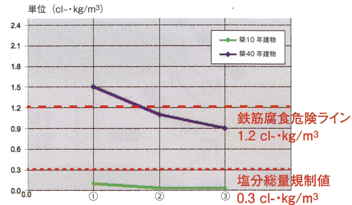
塩分試験測定結果グラフ
