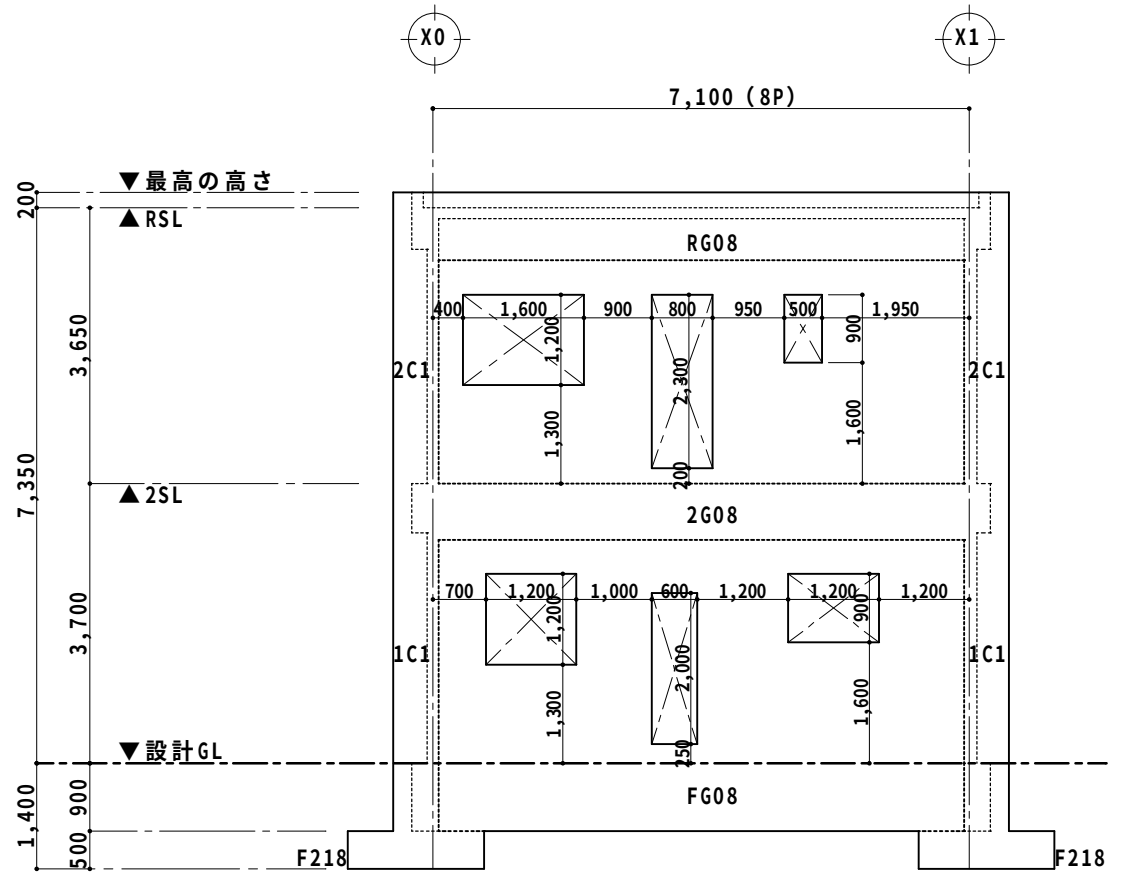
Y 3 軸組図
