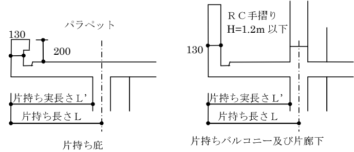
図13－4. 片持ち床スラブの用途
