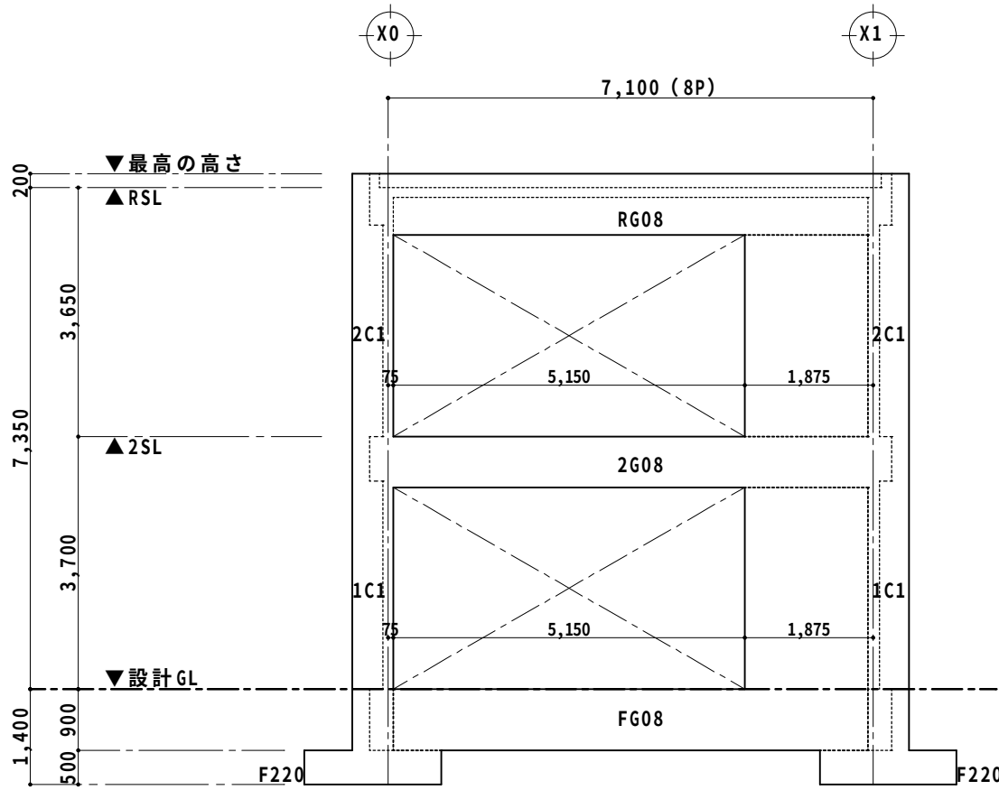
Y 2 軸組図
