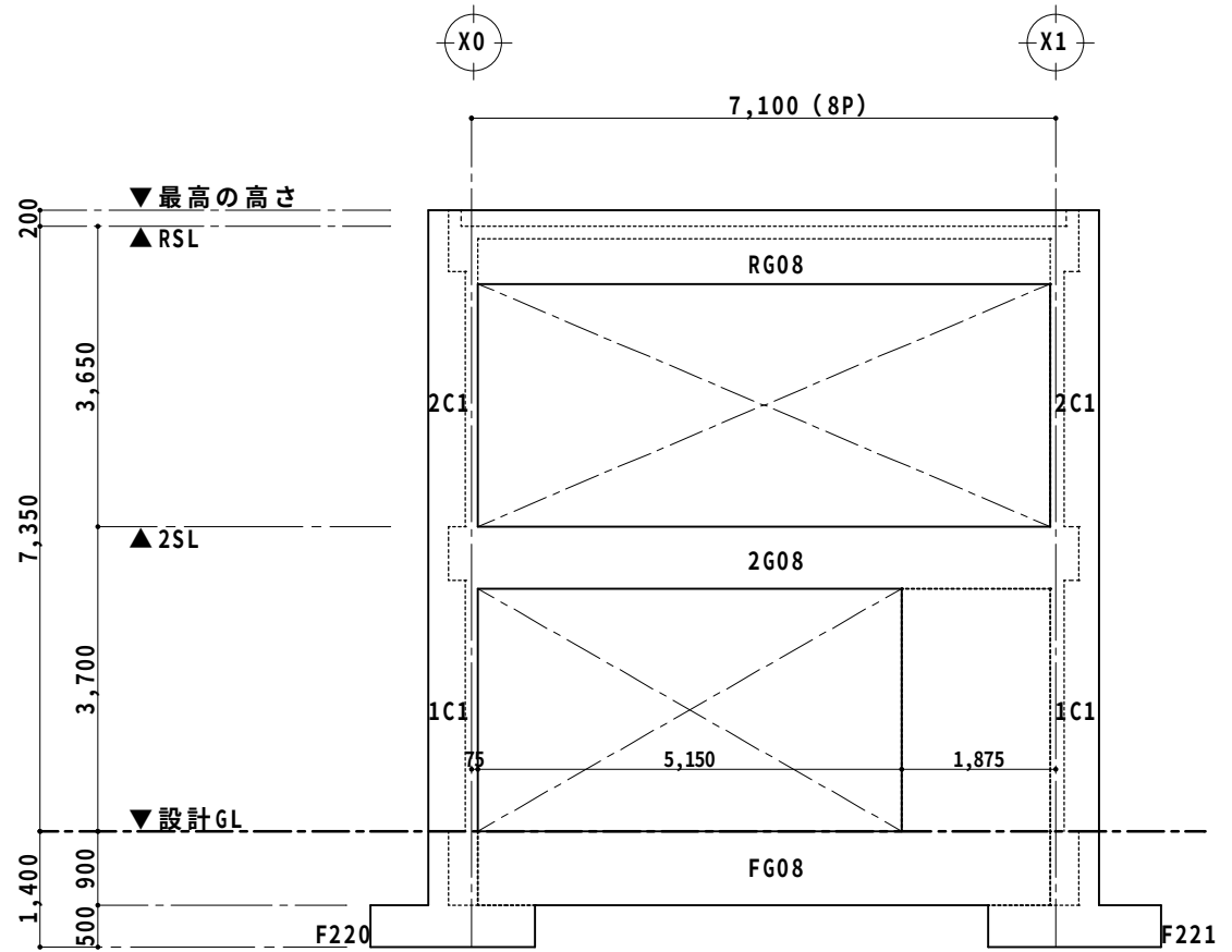
Y 1 軸組図
