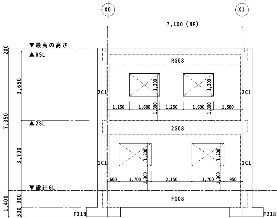
Y 0 軸組図
